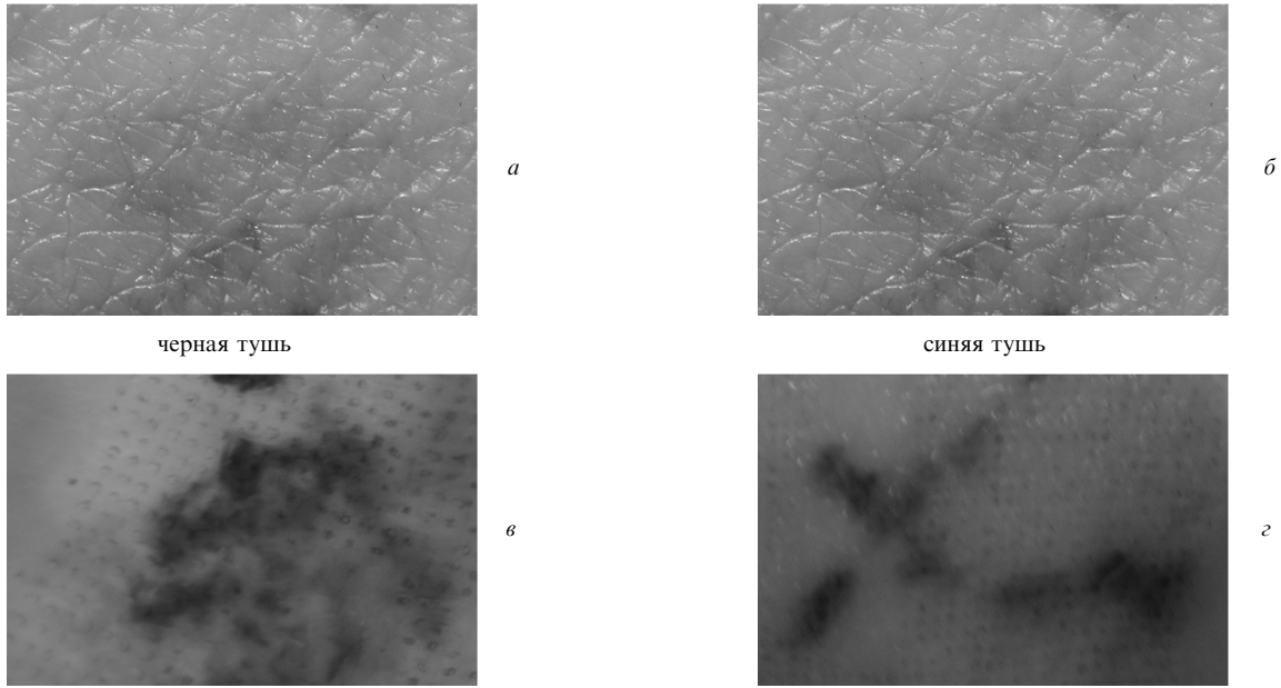
Рис.2. Изображения поверхности кожи с татуировкой черной (а, в) и синей (б, з) тушью; образец с татуировкой до воздействия глицерина (а, б) и после микроперфорирования поверхности и воздействия глицерина в течение 24 часов (в, з).
